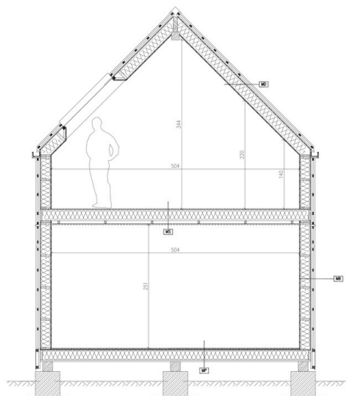
Przekrój roboczy
