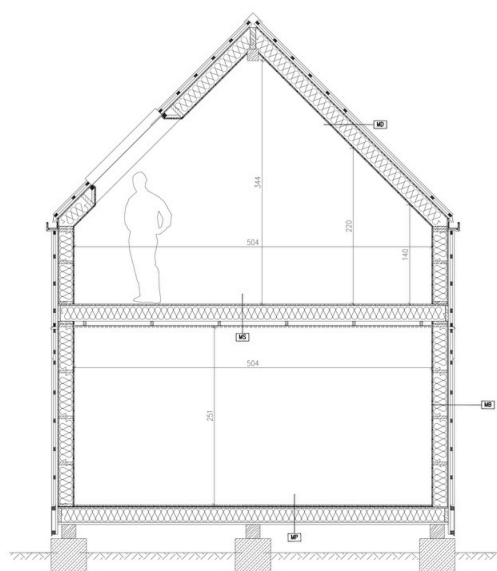
Przekrój roboczy
